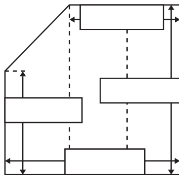
Dachschräge links
